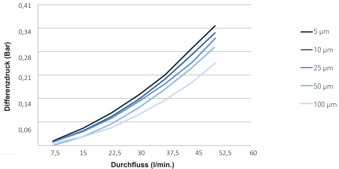
Druckverlust (Bar vs. l/min.)
